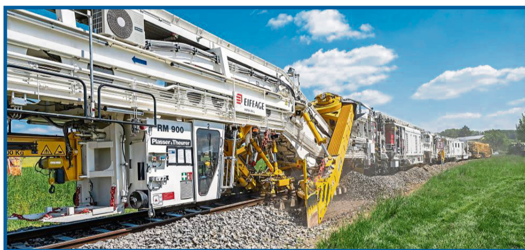
Bis auf 650 Meter Länge kann der Zug „RM 900“ auf den Schienen anwachsen. Der Einsatz der Maschine dürfte nicht nur für Bahnfans ein Highlight sein.
